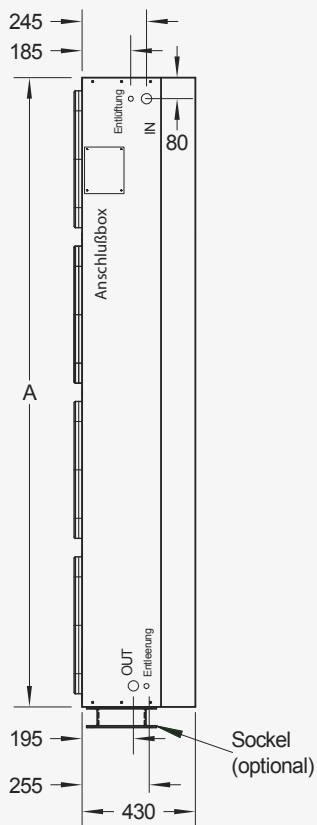
SEITENANSICHT
