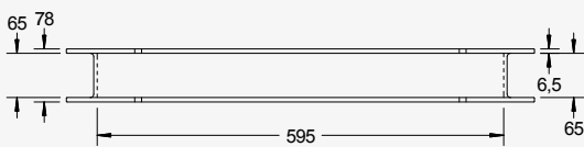
VORDERANSICHT
