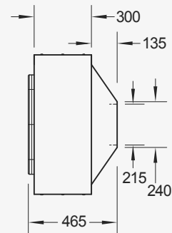
DRAUFSICHT
