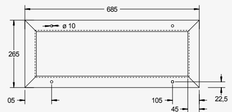
DRAUFSICHT
