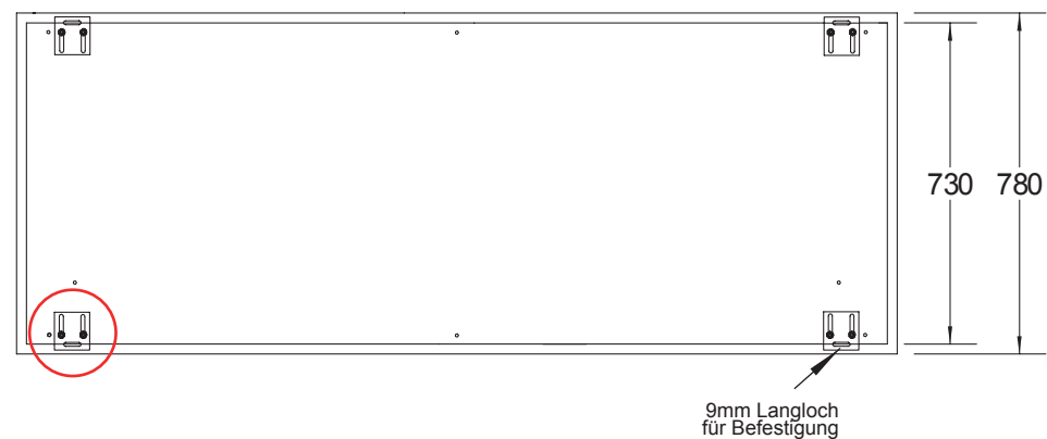
DRAUFSICHT
